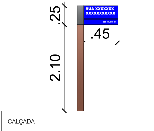
PLACA DE IDENTIFICAÇÃO DA RUA ESC _____ 1/25
