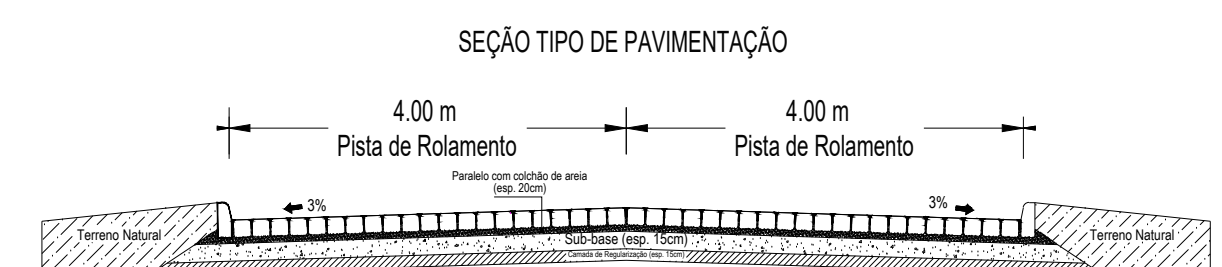
DETALHAMENTO DA SEÇÃO ESCALA 1/125
