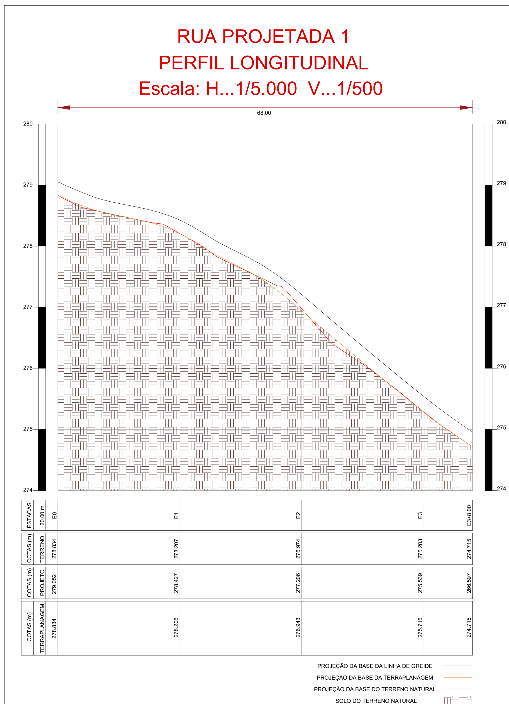
PERFIL LONGITUDINAL ESCALA 1/500
