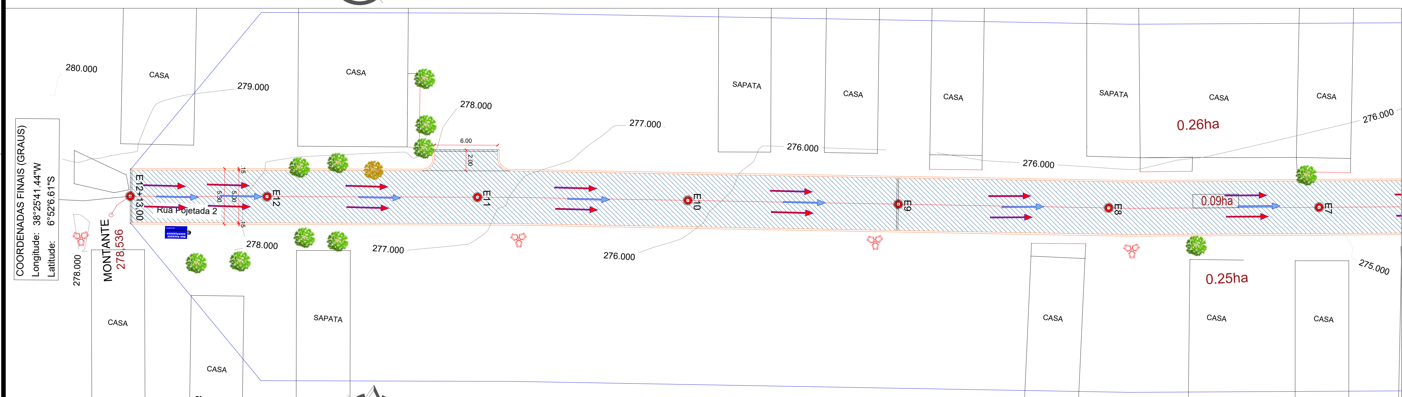
PLANTA DE SITUAÇÃO - GERAL EST. 7 A EST. 12+13,00
