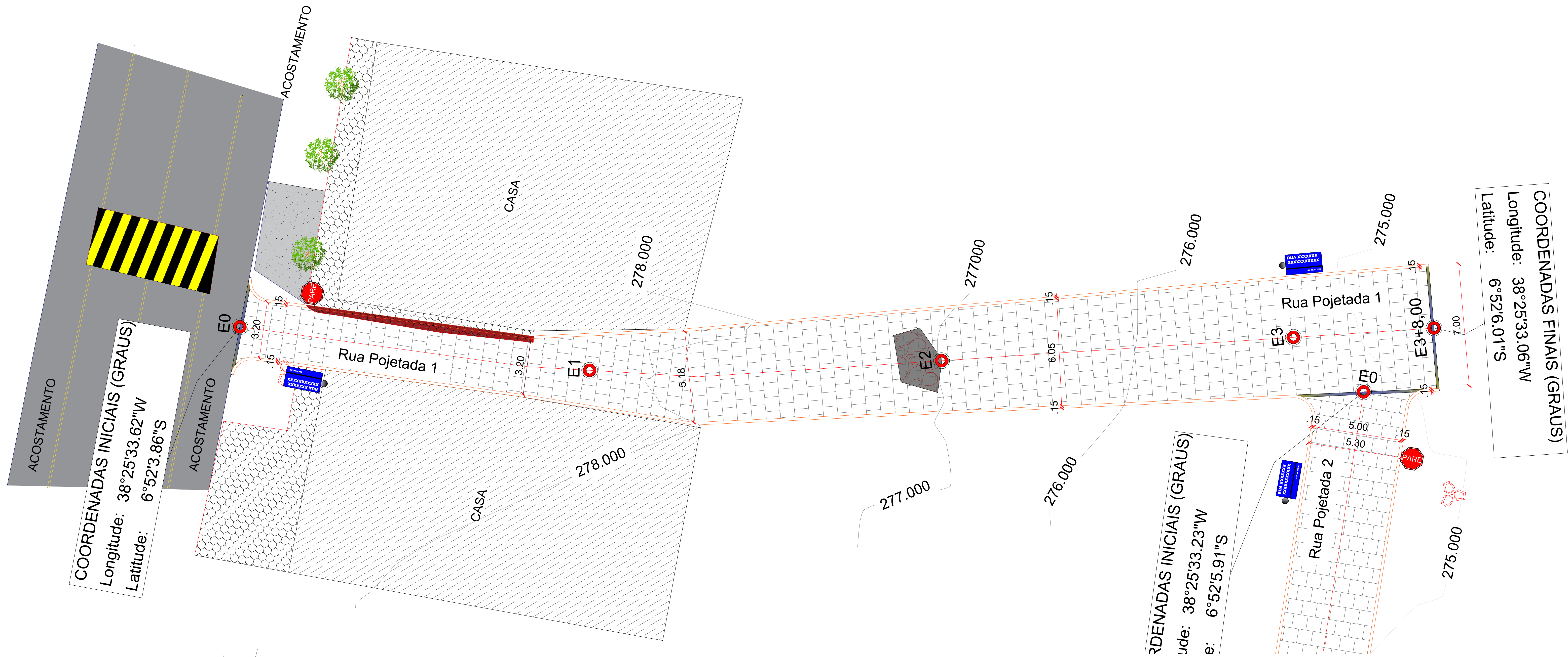
PLANTA DE SITUAÇÃO - GERAL ESCALA 1/150
