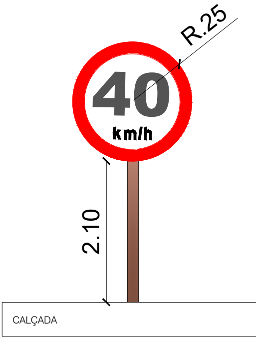
PLACA DE SINALIZAÇÃO ESC _____ SEM ESCALA
