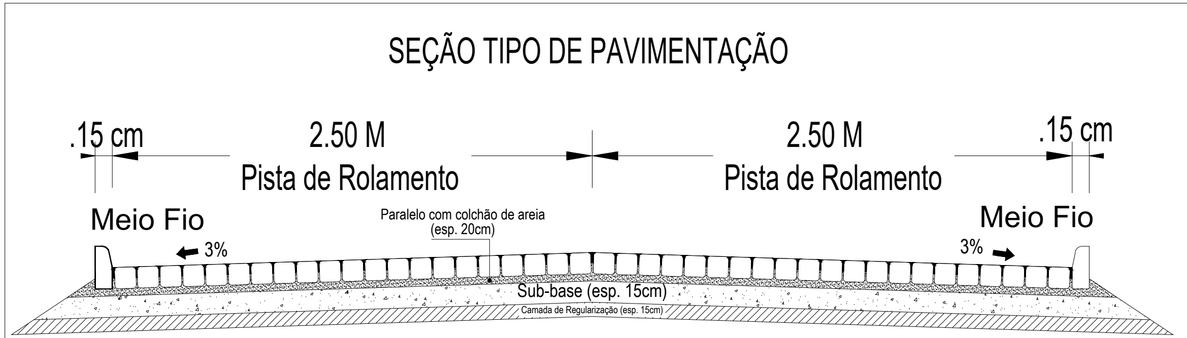
DETALHAMENTO DA SEÇÃO ESCALA 1/75
