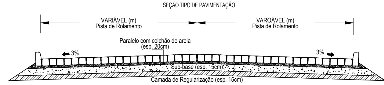
DETALHAMENTO DA SEÇÃO ESCALA 1/100
