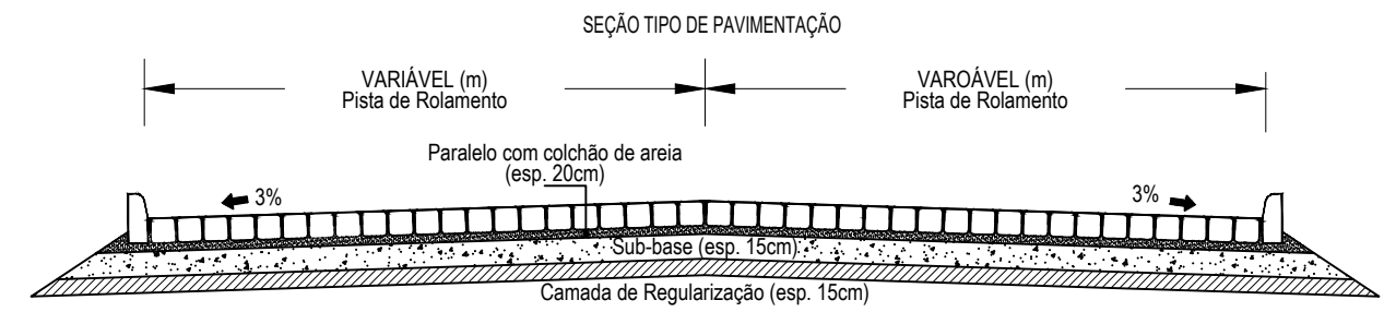
DETALHAMENTO DA SEÇÃO ESCALA 1/100
