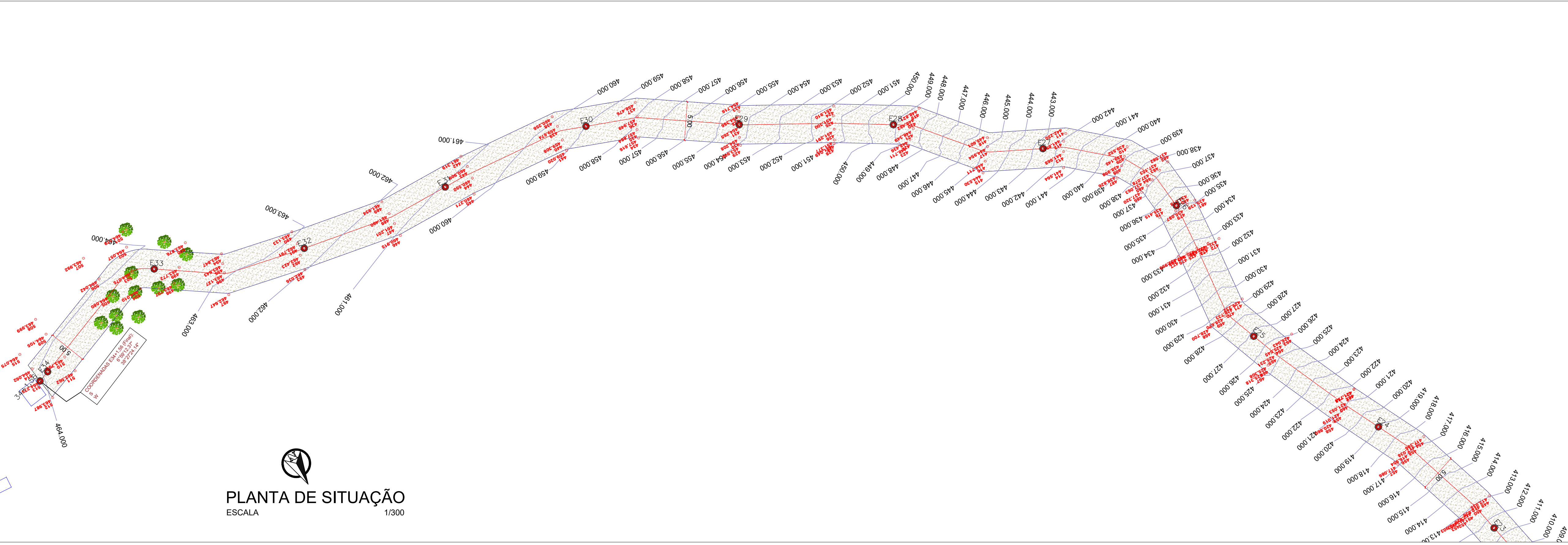
PLANTA DE SITUAÇÃO ESCALA 1/300
